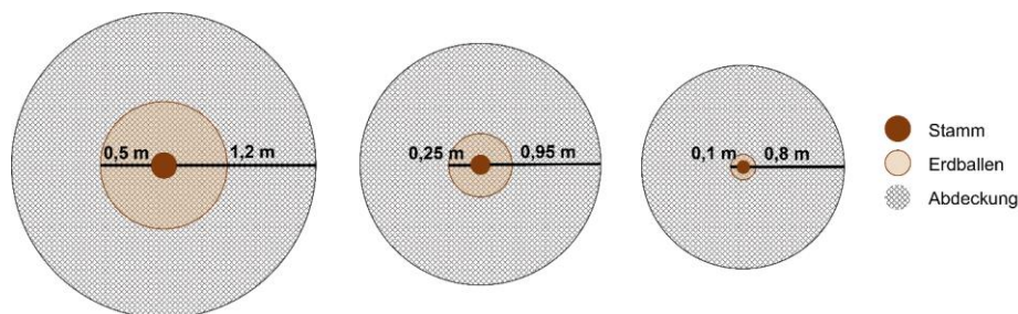
Abbildung 6: Erforderliche Fläche für die Bodenabdeckung abhängig von der Größe der Wurzelballen (Quelle: EPSD, 2025).
